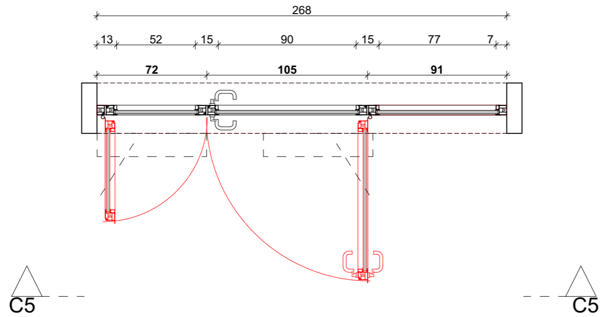
0 Poziom 0 - drzwi_detail -1:25 1:25
